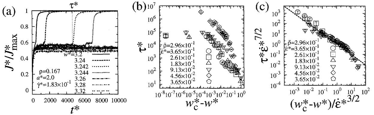
図 1: (a) 規格化された流量 J^*/J_{\max}^* の時間発展. (b) 遷移時刻 \tau^* のボトルネック幅 w^* 依存性. (c) そのスケーリング関数 f(x) .
