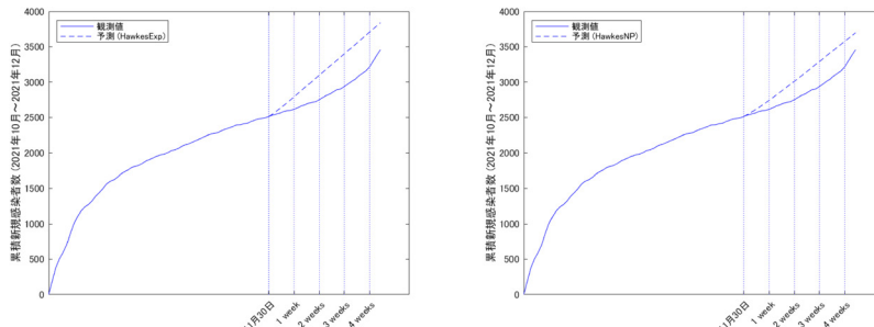
図 5.2 予測月が 12 月のときの累積新規感染者数の予測値と観測値をプロットした。左図がパラメトリック Hawkes モデル、右図がノンパラメトリック Hawkes モデルに関するものである。x 軸の 0 から 11 月 30 日と表示されている点までが学習機関を表す。すなわち、この場合は 10 月 1 日から 11 月 30 日までである。1week, 2weeks, 3weeks, 4weeks と表示されている点はそれぞれ予測月の 7 日、14 日、21 日、28 日を表している。また、グラフの実線は観測値、破線は予測値を表わしている。
