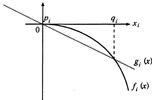
図 3: 線形緩和の例
