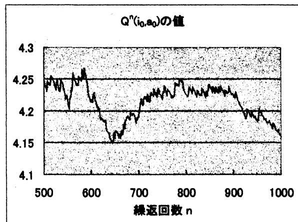
図 1 Q^0(i, a) = 0, \gamma(n) = \frac{1}{1+n} のときの収束
