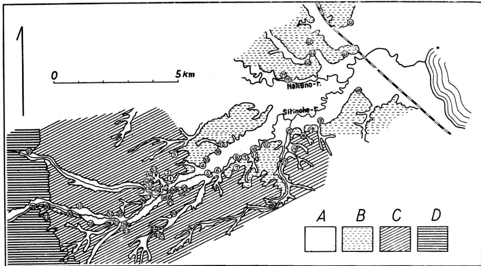
青森縣七戸町近傍地質概念圖 A: 沖積層 B: 七戸層 C: 倉石層 D: 第三系 (番號は實際に觀察を行へる處箇)
