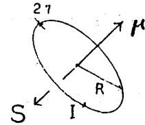
図2. 電子の永久電流モデル。 角運動量ベクトル S と、 磁気能率 \mu の方向は逆平行である。
