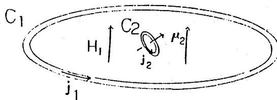
図1. 二つのリング状の超電導体 C_1 , C_2 より成立する系。
