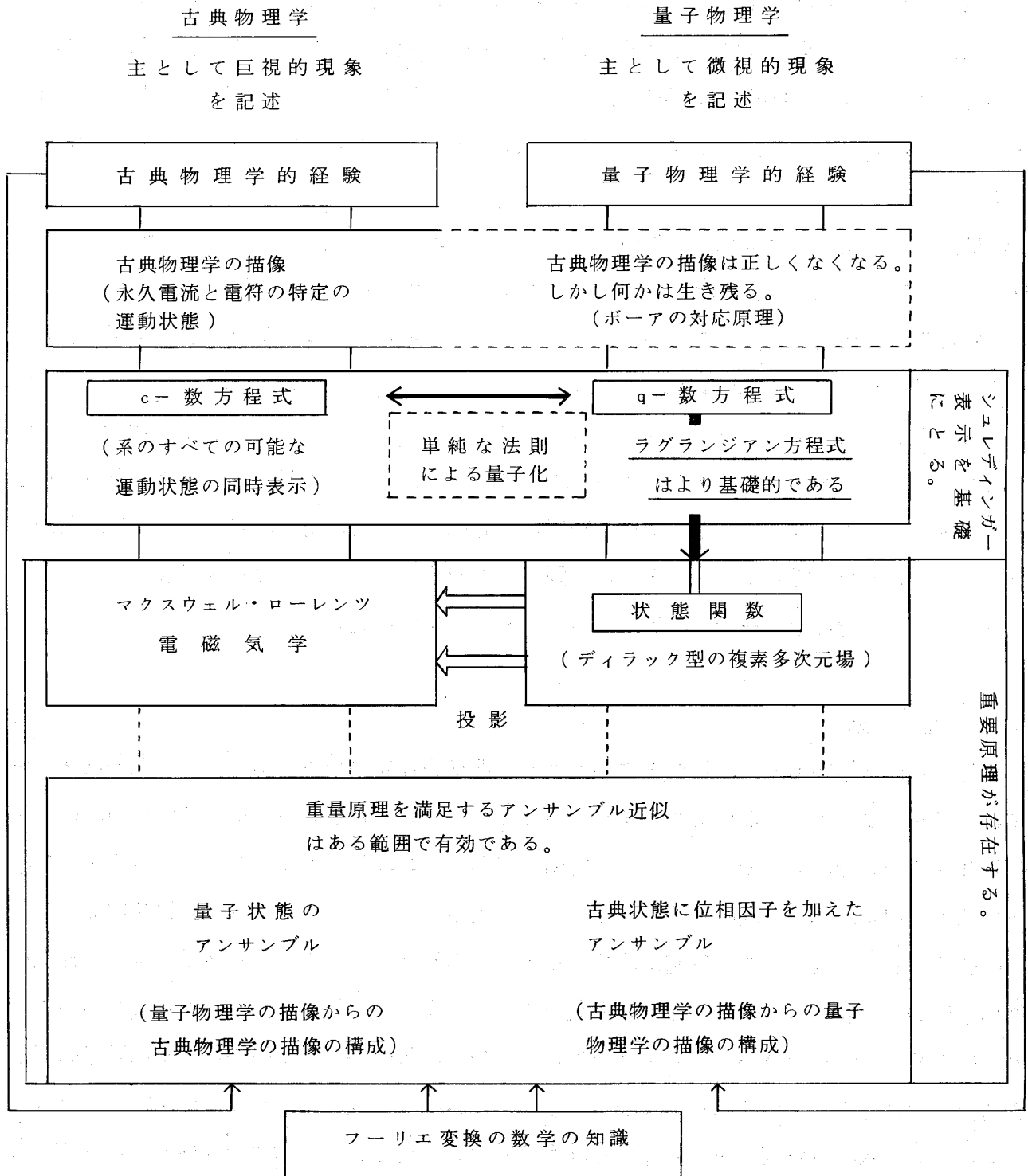
ダイアグラム 1. 新体系物理学の見る 物理学的世界の多重構造
