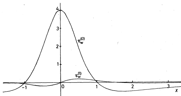
図9 定常流に対する壁面すり忘れ分布 [式 (6.6), (6.7) 参照]。
