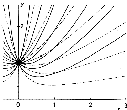
図2. 図1に対する定常 Stokes 流, および定常渦なし流 (破線) の流線. ( \psi は等間隔)
