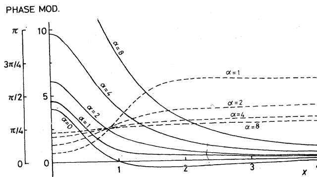
図8. 正弦的に強さの变化する点渦による壁面すり忘れ。実線はその絶対値、破線は位相角を表わす。 \alpha=0 は定常解そのものを示す [式 (6.2) 参照]。
