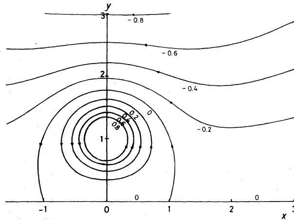
図7. 点 (0, 1) に点渦をおいたときの定常 Stokes 流の流線。流線に付した値は \psi_{st}/c の値 [式 (6.3) 参照]。
