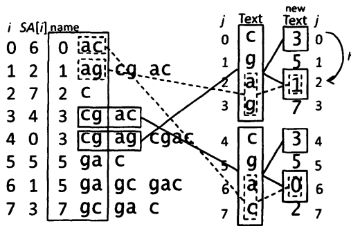
図 2: Doubling
