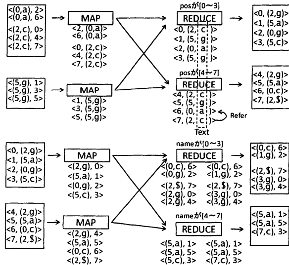
図 5: Tref/Rename
