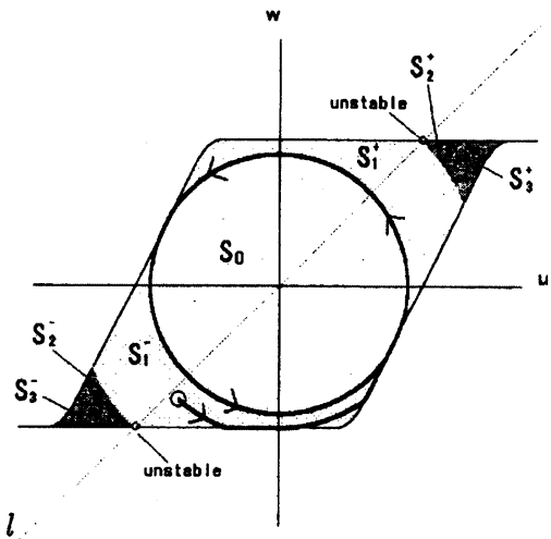
Fig. 6 (u_0, w_0) \in S_1
