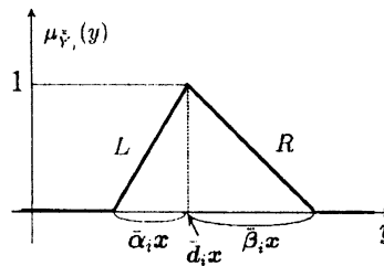
図 2: 目的関数に対応するファジィランダム変数を特性付けるメンバシップ関数 \mu_{\bar{\tilde{Y}}_i}(y) の例
