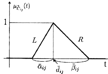
図 1: ファジィランダム変数係数を特性付けるメンバシップ関数
