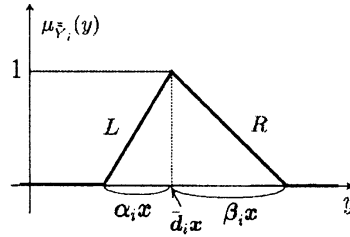
図 4: ファジィランダム変数係数のメンバシップ関数
