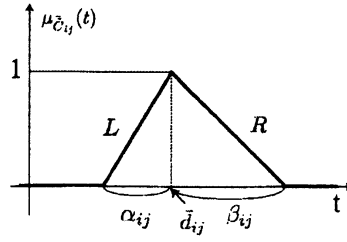
図 4: ファジィランダム変数係数のメンバシップ関数
