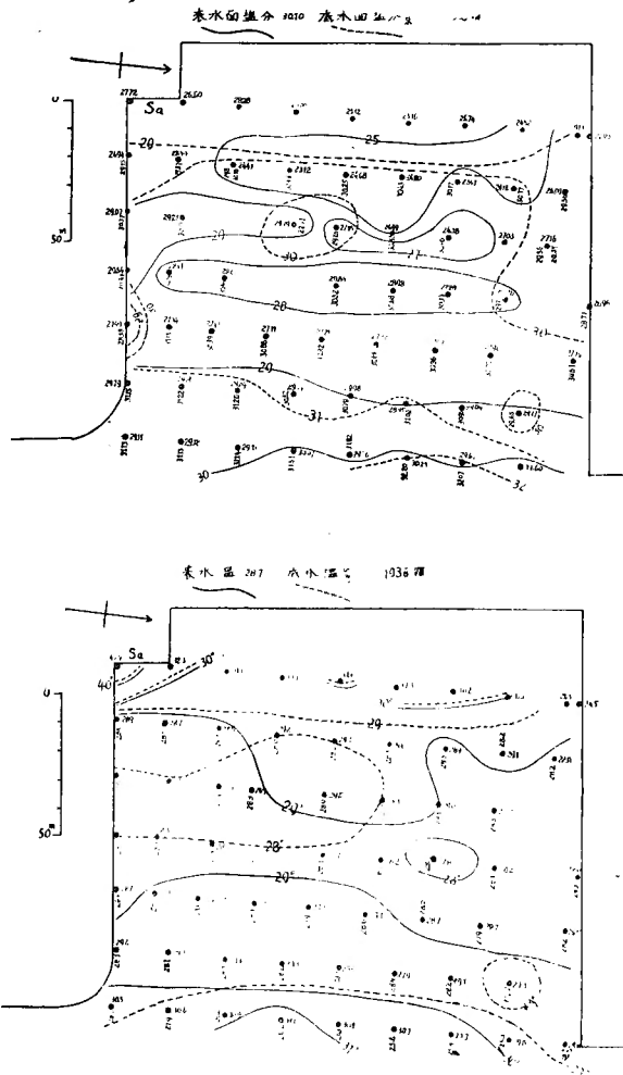
第5圖 別府突堤北側水溫、鹽分分布
