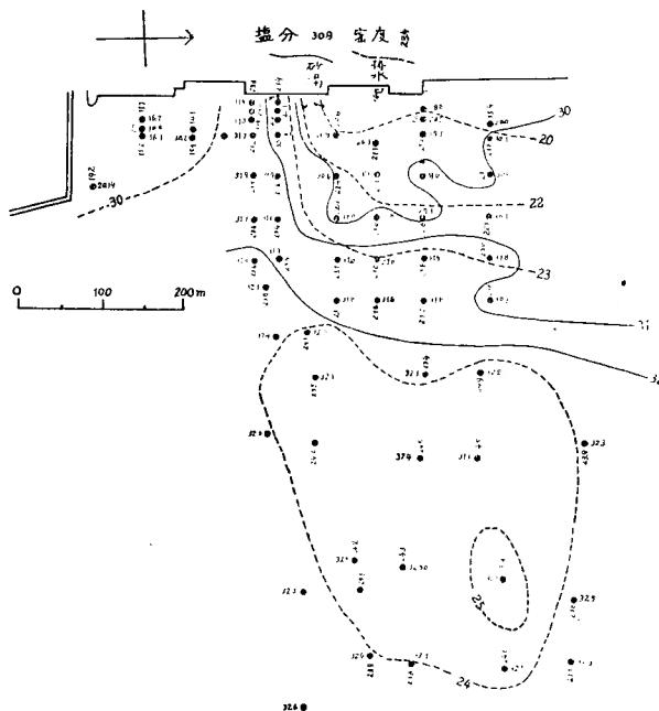
第 7 圖 別府龜川沖底水面鹽分密度分布
