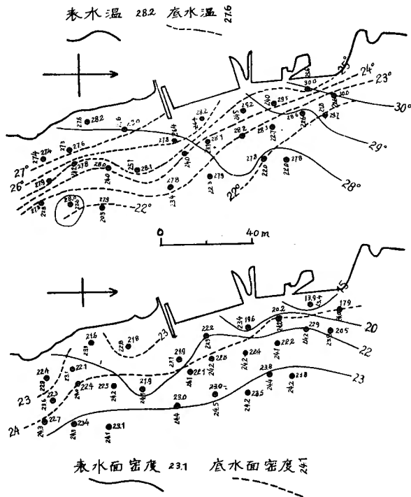
第9圖 龜川沿岸水温、密度分布
