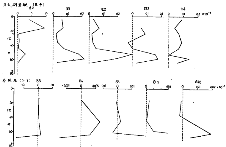
第 14 圖 別府湾深處の垂直安定度夏冬比較
