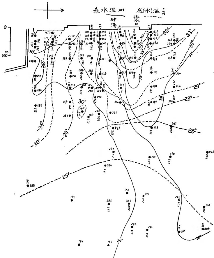
第 6 圖 別府龜川沖温度分布
