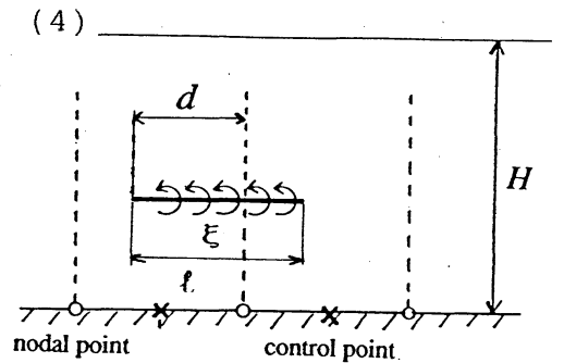
Fig.1. Vortex-sheet element
