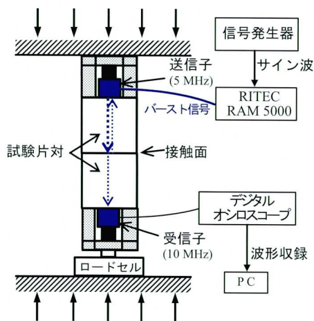
図10 固体接触面におけるパースト波透過測定
