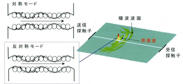
図3 接触界面に沿った超音波伝搬モード
