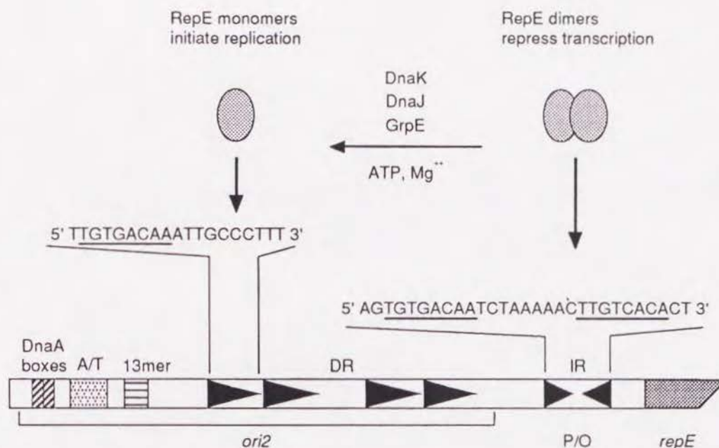
Fig.2 mini-F プラスミドの構造および複製調節のモデル図。複製オリジン ( ori2 ) は、2つの DnaA 蛋白質結合サイト (DnaA boxes), A/T rich region (A/T), 大腸菌複製オリジン oriC の 13mer 配列に似た 13 bp の配列 (13mer), 4つの 19 bp イテロン (direct repeat, DR) からなる。その右隣の repE 遺伝子の プロモーター/オペレーター領域 (P/O) には、inverted repeat (IR) が存在する。DR には RepE モノマーが、IR にはダイマーが結合し (Ishiai et al. , 1994)、それぞれ DNA 複製開始および repE 遺伝子の転写抑制を行う。1つ目のイテロンと、IR の塩基配列を示した。下線は両者に共通する 8 bp 配列である。
