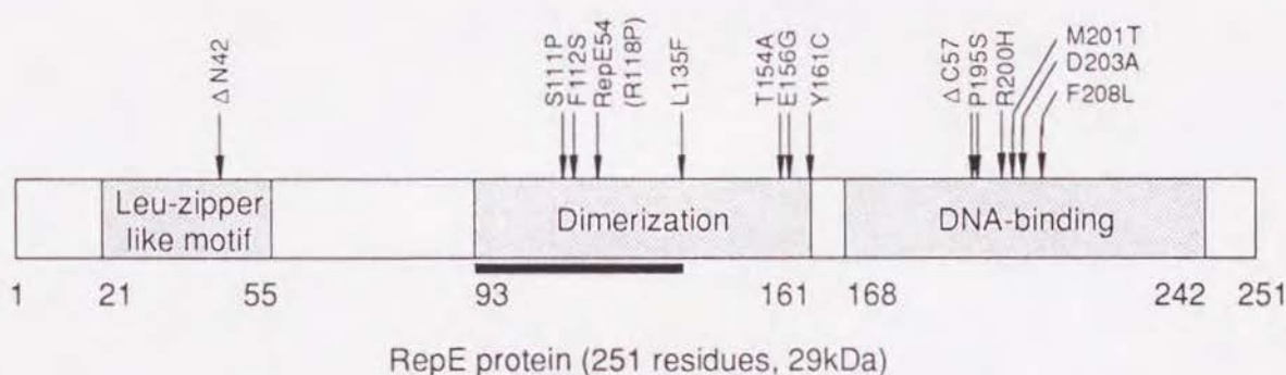
Fig. 16 RepE 蛋白質の機能構造モデル。リプレッサー活性欠損変異体 (R118 を含む) のアミノ酸置換部位と欠失変異 NΔ42 および CΔ57 の末端の位置を示した。黒いバーは以前シャペロン要求性なくなったコピー・アップ変異が分離された領域である。ロイシンジッパー様配列および、ダイマー形成と DNA 結合にかかわると考えられる領域の位置を影付きの四角で示した。
