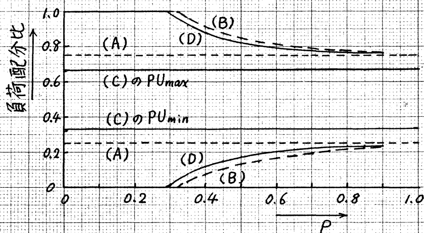
図9. 負荷配分比特性 ( C_{min}:C_{max}=1:3 )
