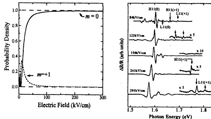
図1: 単一ミニバンド構造を仮定した電子波動関数の存在確率の電場依存性 図2: 異なる電場における ER スペクトル
