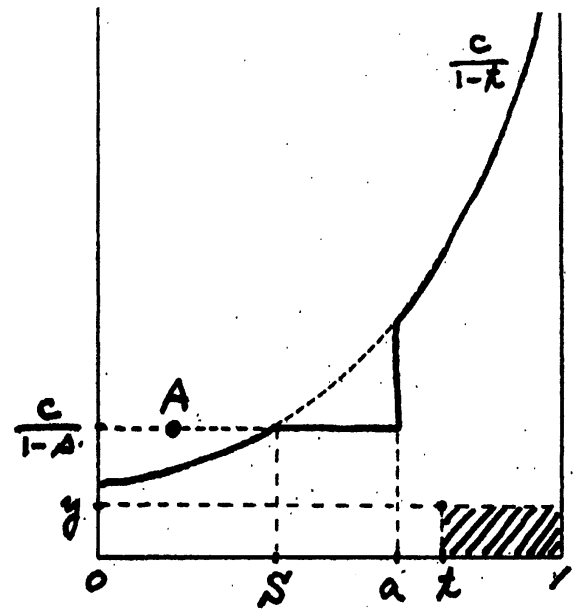
Case (2b): x \geq a, 0 \leq y < \frac{c}{1-a}
