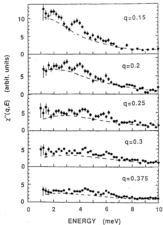
第3図 \text{RbMn}_{0.39}\text{Mg}_{0.61}\text{F}_3 ( T_N=19\text{K} )の T=4.5\text{K} でのエネルギースペクトルの波数依存性 ( q=0.15, q=0.2, q=0.25, q=0.3, q=0.375 )。 10) イジングクラスター励起から生じるピークがオーバーダンプした幅広いスペクトル(破線)の上に重なっている。
