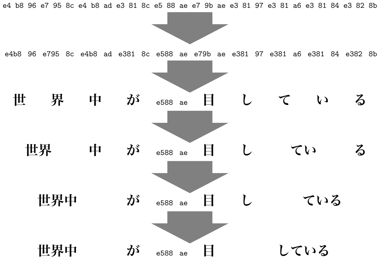
図 5: yellowback/gpt-neo-japanese-1.3B のトークナイザ動作概要
