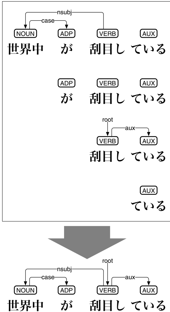
図 3: UD 係り受けリンクの抽出と組み上げ
