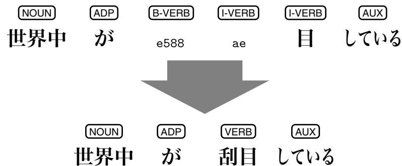
図 4: yellowback/gpt-neo-japanese-1.3B における UD 品詞付与と組み上げ
