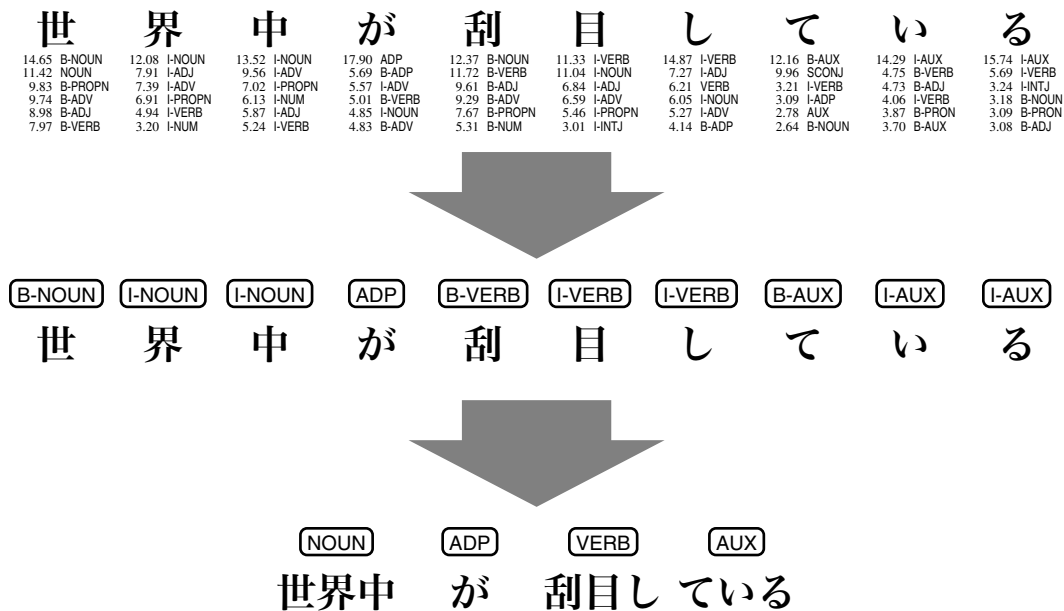
図 2: 単文字トークナイザにおける国語研長単位 UD 品詞付与と組み上げ
