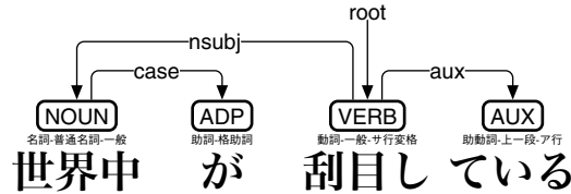
図 1: 国語研長単位 UD の CoNLL-U と deplacy による可視化
