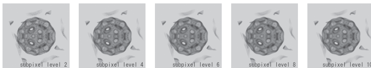
図9 サブピクセルレベルの変化にともなう画質の変化 (フラーレン分子の電子密度分布、要素タイプ：四面体、要素数：1,250,235)
