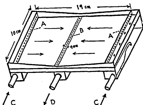
第2図 Olfactometer
