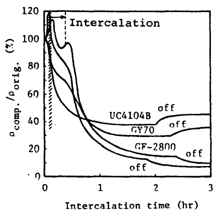
Fig. 1 K 層入に伴う電気抵抗率変化 ( \rho_{\text{orig.}} , \rho_{\text{comp.}} : 原試料および K intercalation の電気抵抗率)
