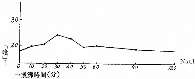
第 2 圖 各煮沸時間ト被喰菌數 菌 1 トノ關係
