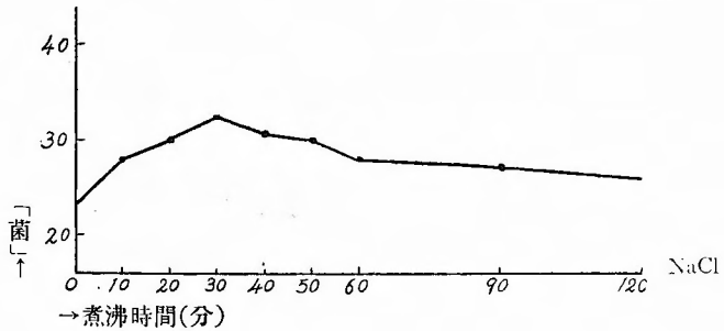
第 2 圖 各煮沸時間ト被喰菌數 菌 1 トノ關係
