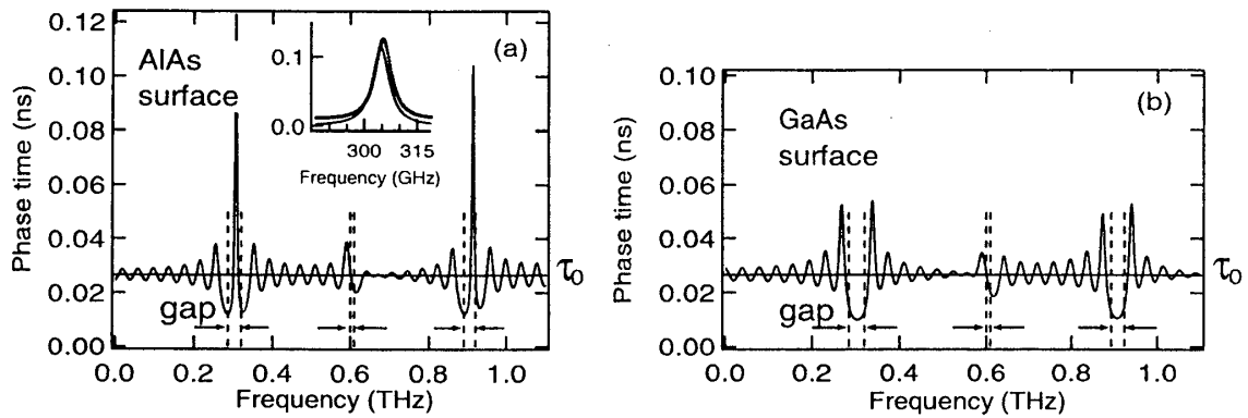
図 14: 位相時間
