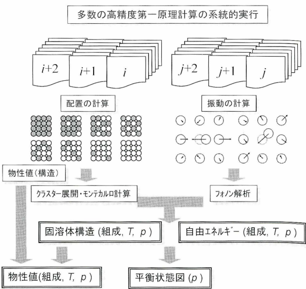
図1 多数の高精度第一原理計算を系統的に実行することで、物質の構造や物性を温度や圧力の関数として系統的に予測するスキーム。
