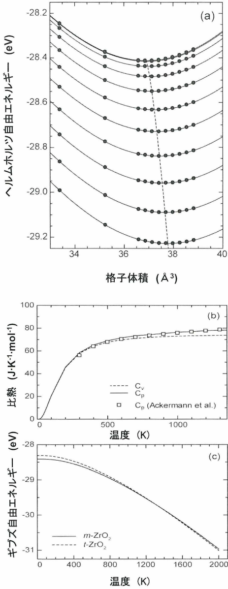
図2 (a)単斜晶 ZrO 2 のヘルムホルツ自由エネルギーを 11 種類の体積と 11 種類の温度 (0-1000K の範囲で 100K 毎) について計算した結果. (b)単斜晶 ZrO 2 の比熱の計算結果と実験結果 7) の比較. (c)単斜晶と正方晶 ZrO 2 のギブズ自由エネルギーの比較.
