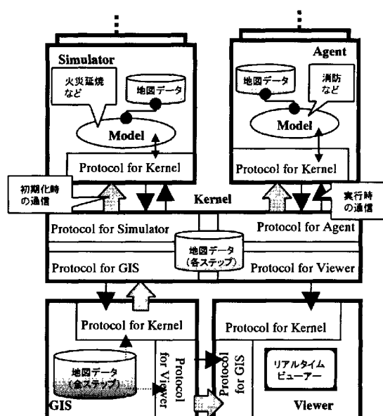
Fig. 3 RoboCup-Rescue Simulator
