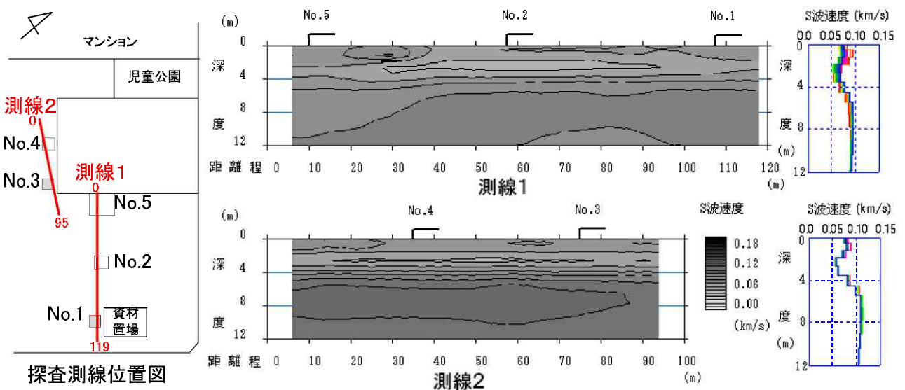
図-3 2次元表面波探索測線位置図と S 波速度断面図ならびに 1次元 S 波速度分布図
