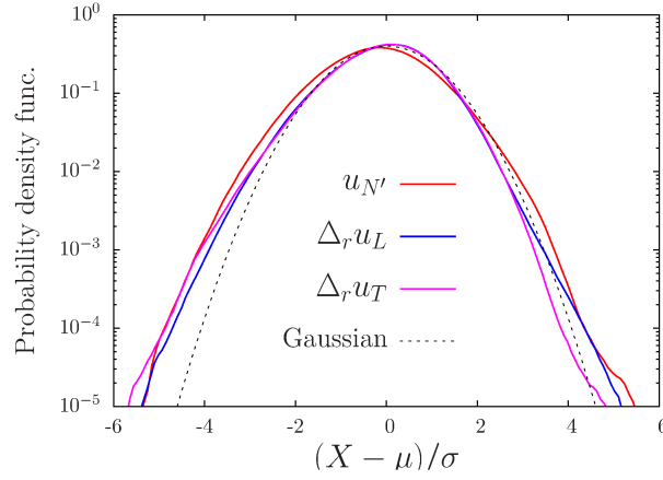
図 2: L, T 成分の速度差と N' 成分の確率分布関数 (参考のために Gauss 分布も示す)。この図では 2 地点差が r = 0.70 であり、慣性領域内のスケールである。また、分布関数は平均がゼロ、分散が 1 になるように規格化されている。
