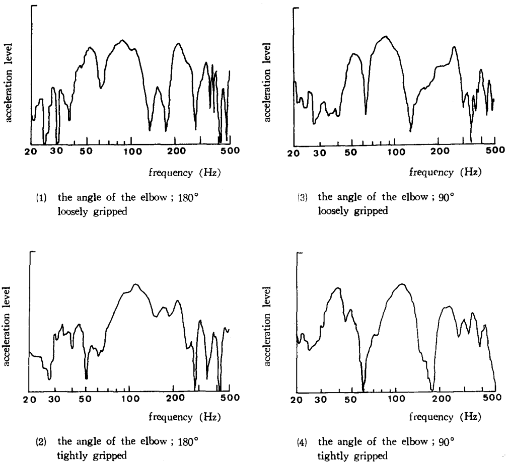
図—1. 片手保持方法とチェーンソーハンドルバー部の固有振動との関係 —被験者A 1 について—
