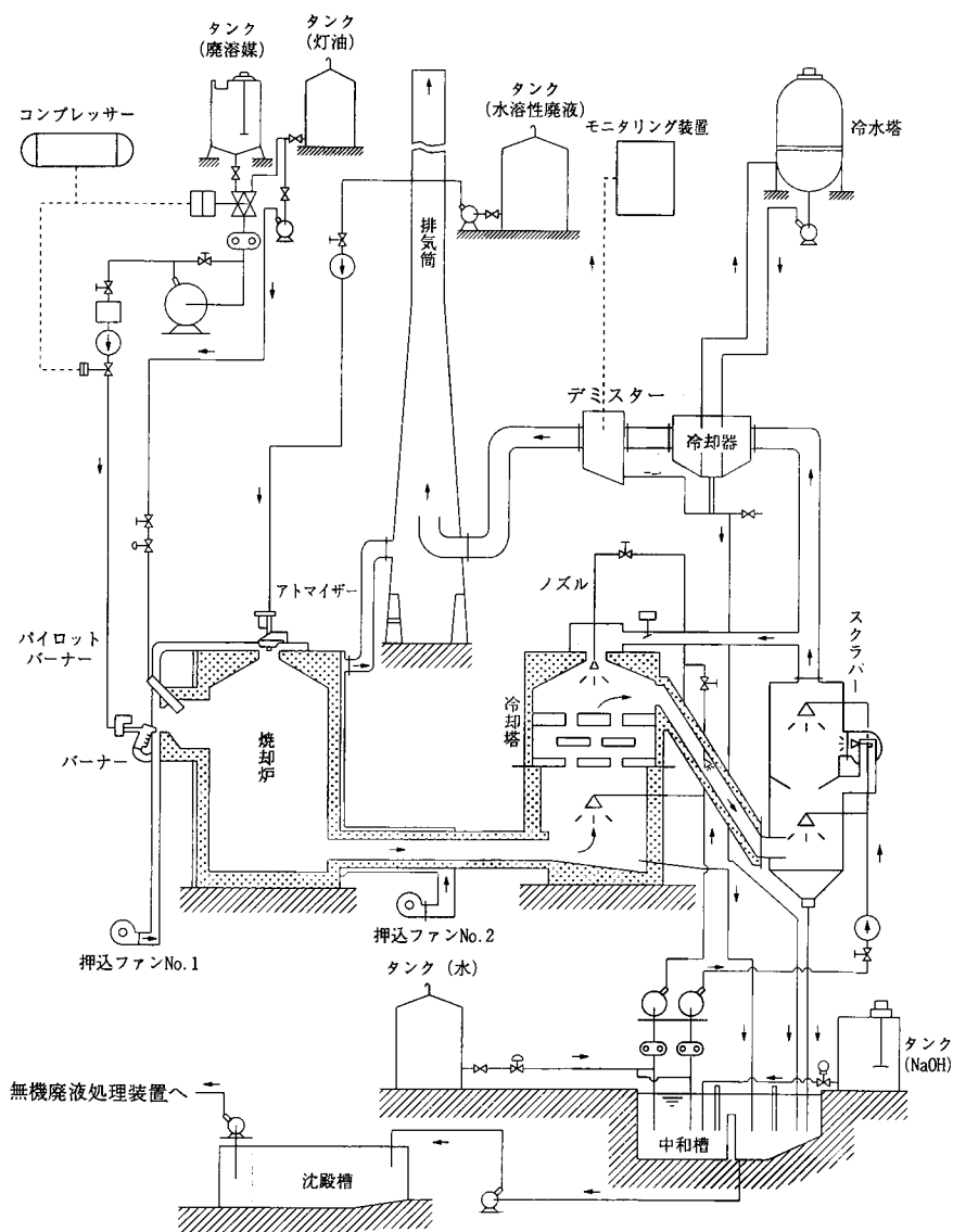
図35-3 KYU(京都大学有機廃液処理装置)のフローチャート
