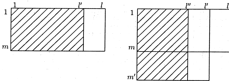
図 2. 漸近的ランダム性の近似的実現
