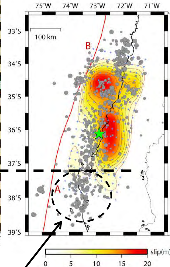
遠地実体波による断層モデル
