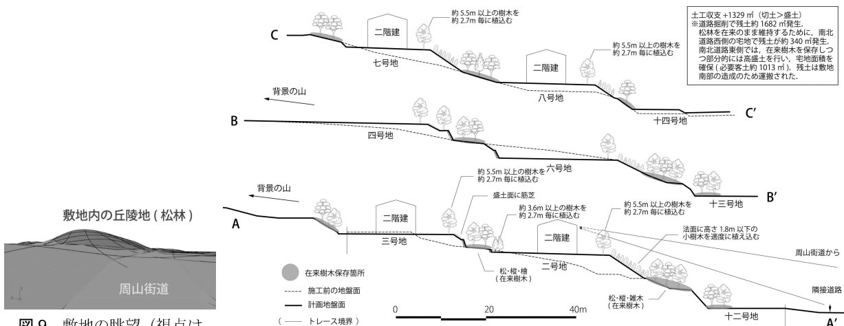
図-10 断面図 (原図をトレースし, 縦横比率を 2:1 から 1:1 に変更, 樹木などを加筆)
