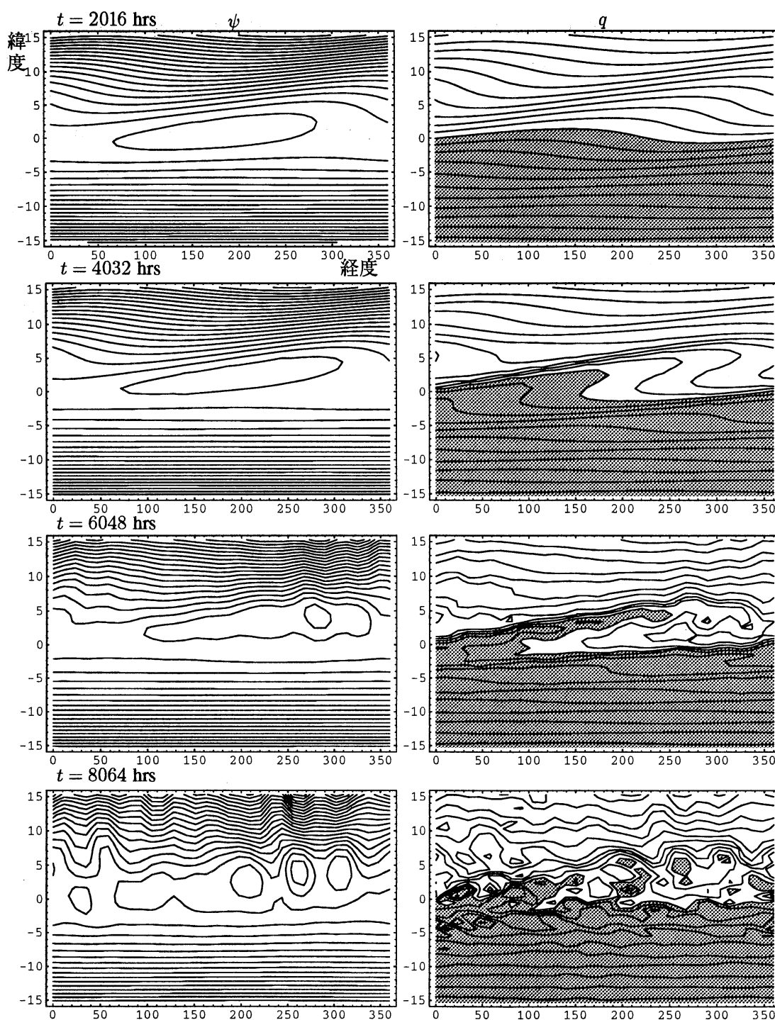
図6 非線型モデルにおける臨界層の時間発展
