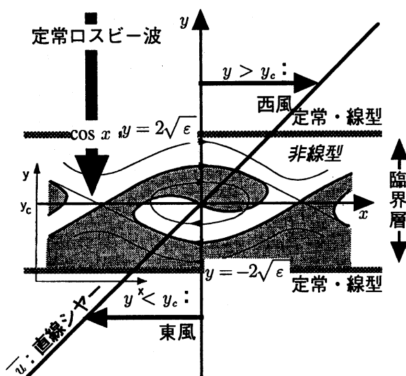
図1 非線型臨界層のモデル (Stewartson, 1978; Warn and Warn, 1978) 細実線: \Psi_0 , Q < 0 に陰影.
