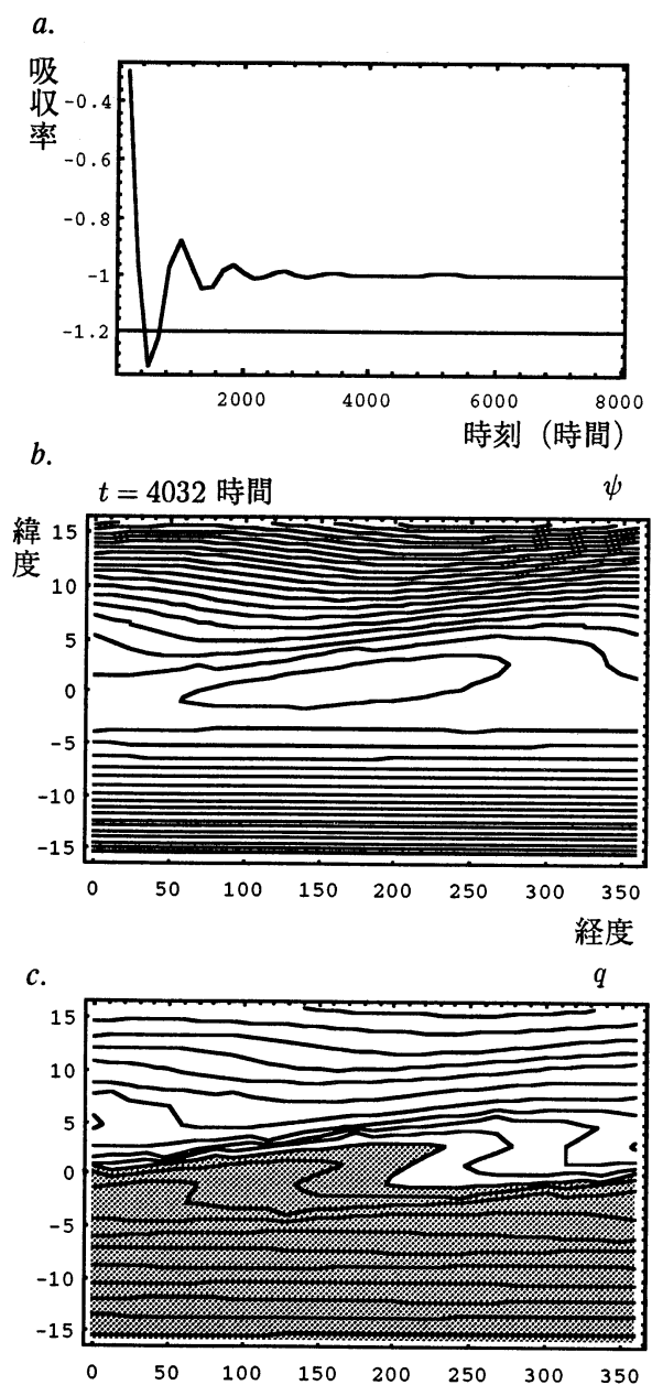
図4 線型モデルでの \alpha (a), \psi (b), q (c)
