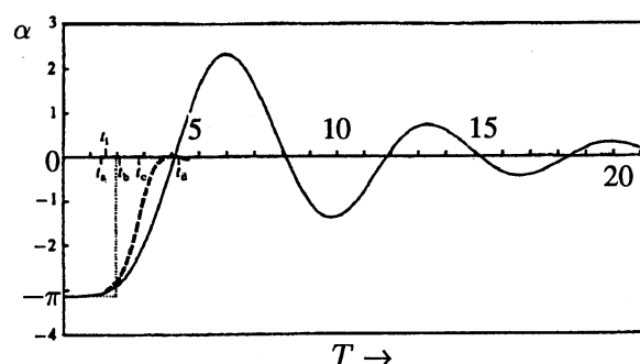
図2 非線型臨界層における吸収率 \alpha の時間発展 (Killworth and McIntyre, 1985).
