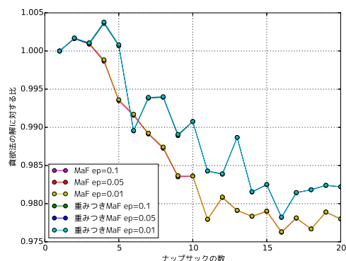
図 10 さまざまな \epsilon に対する Match-and-FPTAS の貪欲法との比 ( k_{\min} = 5 の場合)
