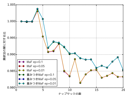
図 9 さまざまな \epsilon に対する Match-and-FPTAS の貪欲法との比 ( k_{\min} = 1 の場合)
