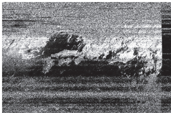
図4 中京大学豊田キャンパスにおいて取得したNOAA-15衛星の気象画像：(a) 本実習で学生が取得したものと、(b) 予備実験で指導教員が取得したもの。両画像は雲と陸地が視認出来る範囲を抽出した。
