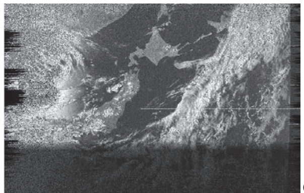
図4 中京大学豊田キャンパスにおいて取得したNOAA-15衛星の気象画像：(a) 本実習で学生が取得したものと、(b) 予備実験で指導教員が取得したもの。両画像は雲と陸地が視認出来る範囲を抽出した。
