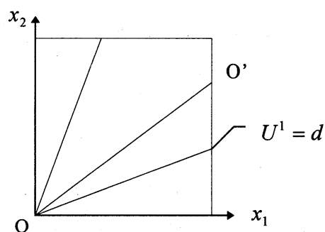
図 3 : (S_1 \times S_2, \text{inddom}) の安定集合
