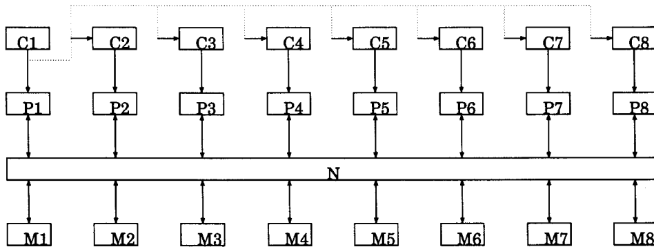
Fig. 5 MIMD Microprocessors, (C : Control Unit ; P : Processor ; N : Organization Network ; M : Memory).
