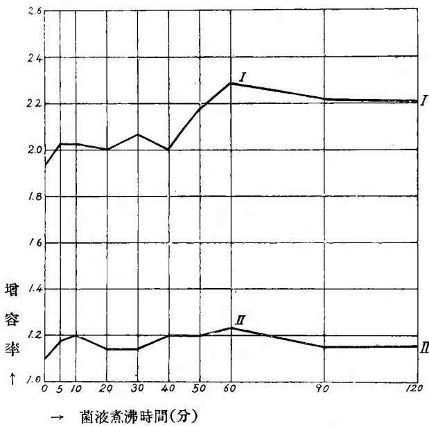
第 1 圖 腸チフス菌煮沸時間ト増容反應 (第3表並ニ第5表參照)
