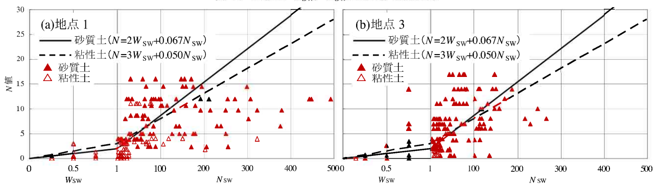
図-3 同一深度における N 値と W_{sw} , N_{sw} の関係
