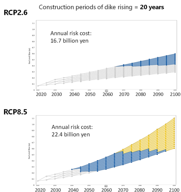
図：堤防嵩上の最適計画
