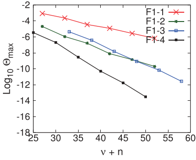
レゾルベントを1つ用いたフィルタ
