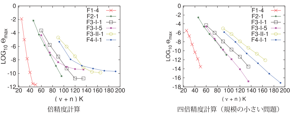
図 27: Chebyshev 多項式の次数の和 \nu + n とレゾルベントの数 K の積 vs. 最大の相対残差の大きさ
