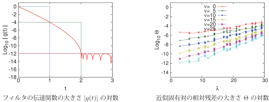
図 2: フィルタ F1-1 ( n = 27 , \mu = 2.0 , g_s = 1\text{E-}12 , g_p = 1\text{E-}4 )
