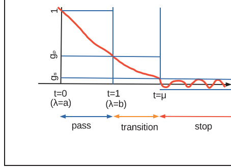
図 1: 伝達関数 g(t) \equiv f(\lambda) の概形
