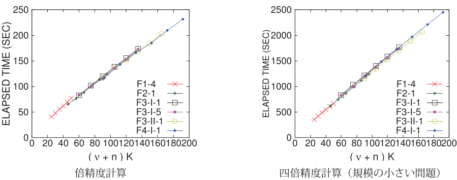
図 28: Chebyshev 多項式の次数の和 \nu + n とレゾルベントの数 K の積 vs. 対角化完了までの経過時間
