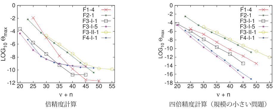
図 26: Chebyshev 多項式の次数の和 \nu + n vs. 最大の相対残差の大きさ
