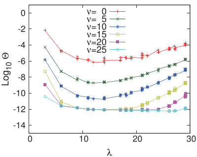
近似固有対の相対残差の大きさ \Theta の対数
