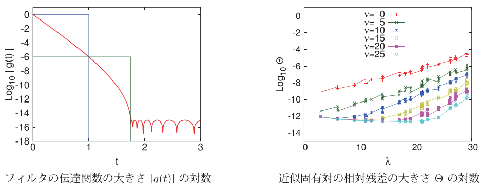
図 3: フィルタ F1-2 ( n = 28 , \mu = 1.75 , g_s = 1\text{E-}15 , g_p = 1\text{E-}6 )
