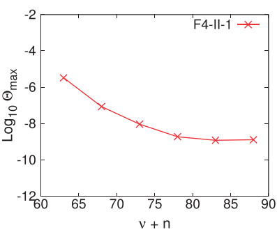
レゾルベントを4つ用いたフィルタ (方式II)
