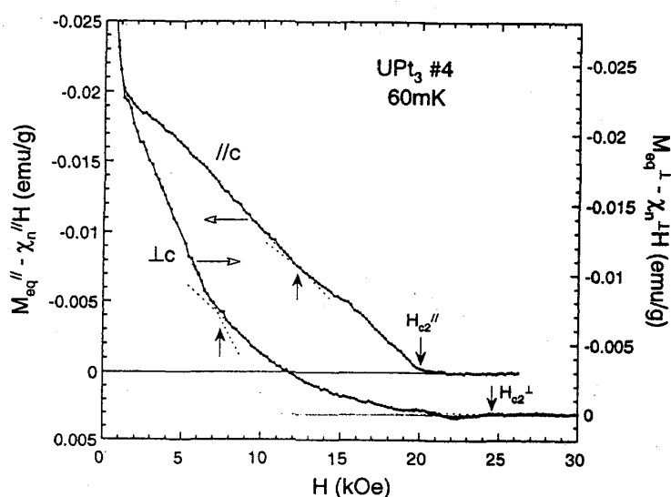
図2 超伝導磁化の磁場依存性
