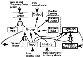
Figure 4.6: Actual Grouping Module.
