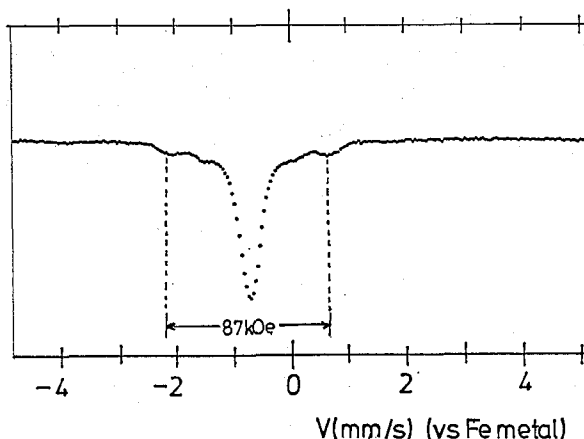
Fig. 4. Mössbauer spectrum of \text{K}_2\text{Sr}(\text{FeO}_4)_2 at 2K
