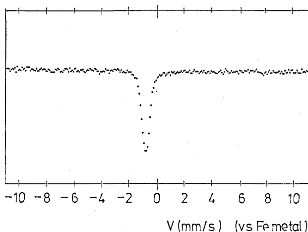
Fig. 3. Mössbauer spectrum of K_2Sr(FeO_4)_2 at 4.8K.
