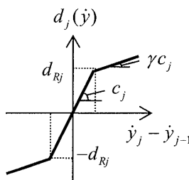
図1 ダンパー復元力特性
