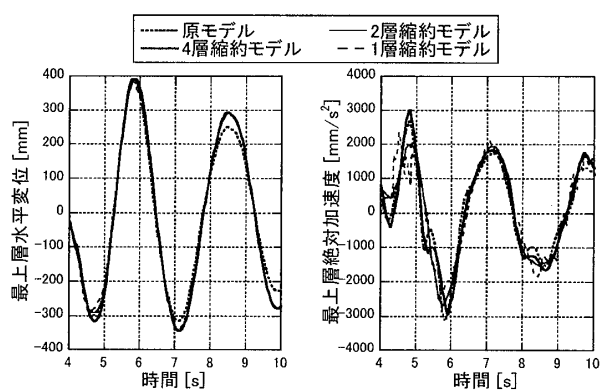
図4 時刻歴応答波形
