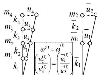
図2 原モデル(左)と縮約モデル(右)
