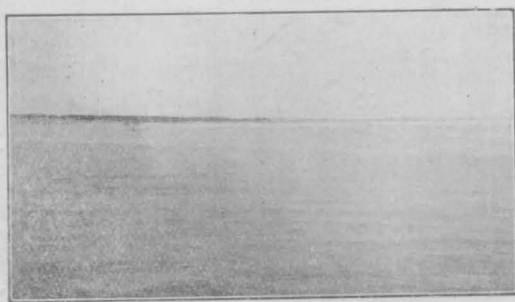
海上から見たスエーデンの準平原地形
