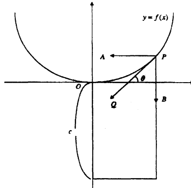
図 1：一般カテナリー曲線
