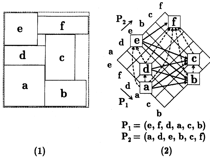
図 1: シーケンス・ペアによる矩形配置表現。(1) シーケンス・ペア, (2) 矩形配置。
