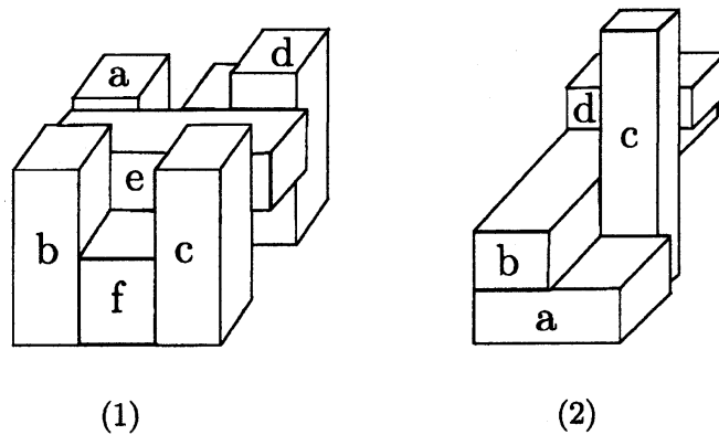
図 2: Sequence-triplet で表現できない直方体配置。
