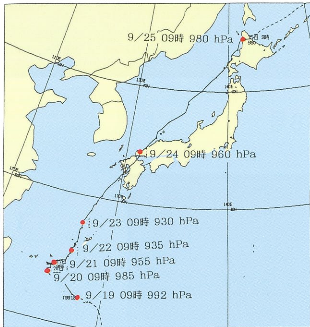
図1 台風9918号の経路と中心気圧
