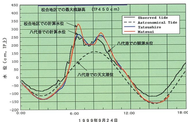
図3 八代港で観測された潮位
