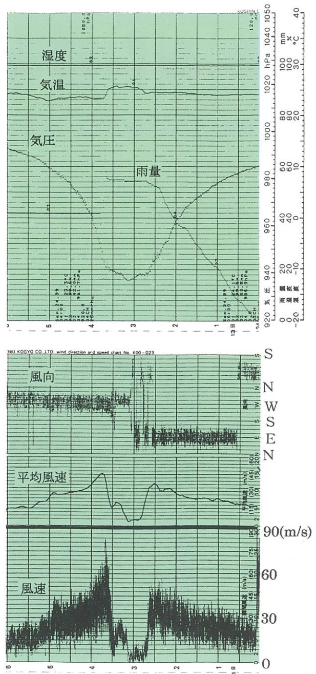
図2 下甕島での気象記録
