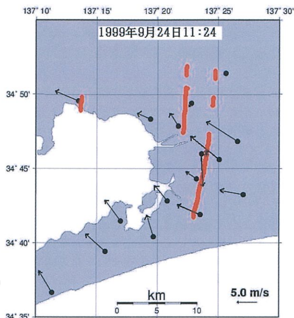
竜巻の通過経路。矢印は観測された地上風の例。この時刻に竜巻は豊橋市役所の東を通過した。
